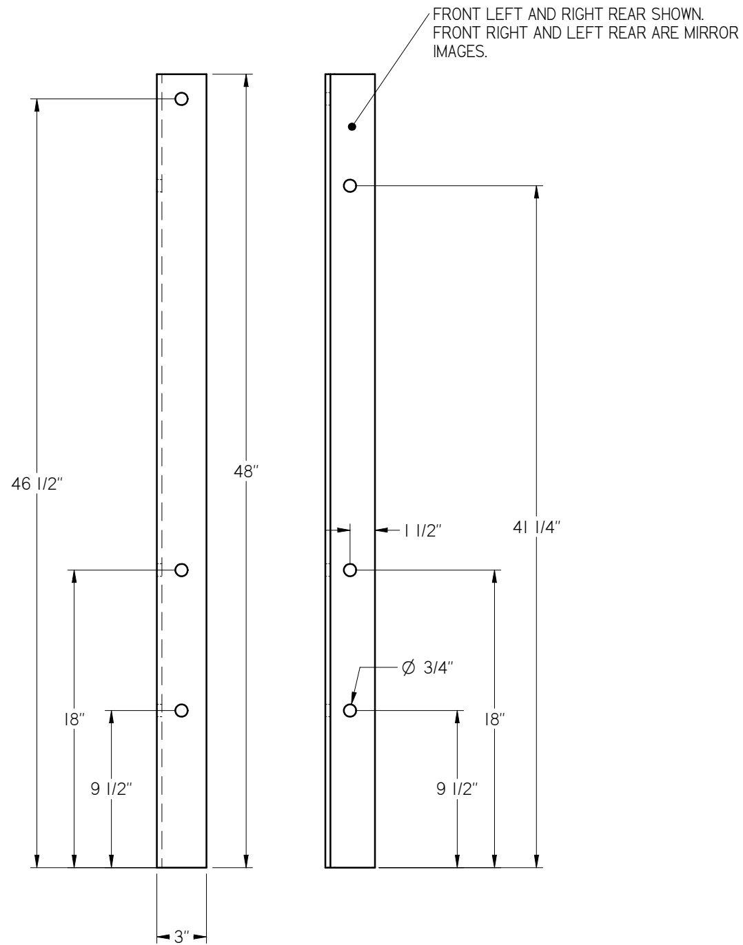
3X3X5/16 ANGLE
